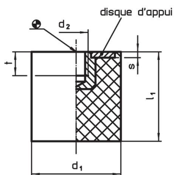
croquis 1
