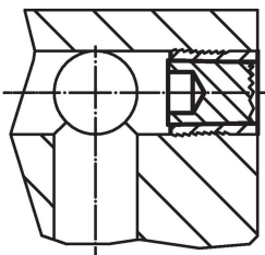
Pression de fonctionnement et de test pour bouchons d'étanchéité à expansion Expander® à tirant
