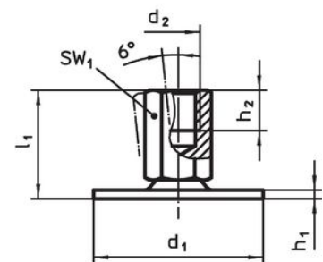
croquis 3
